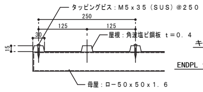
屋根詳細図 1/5
