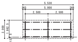
小屋伏図 1/100
