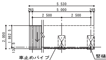
平面図・屋根伏図 1/100
