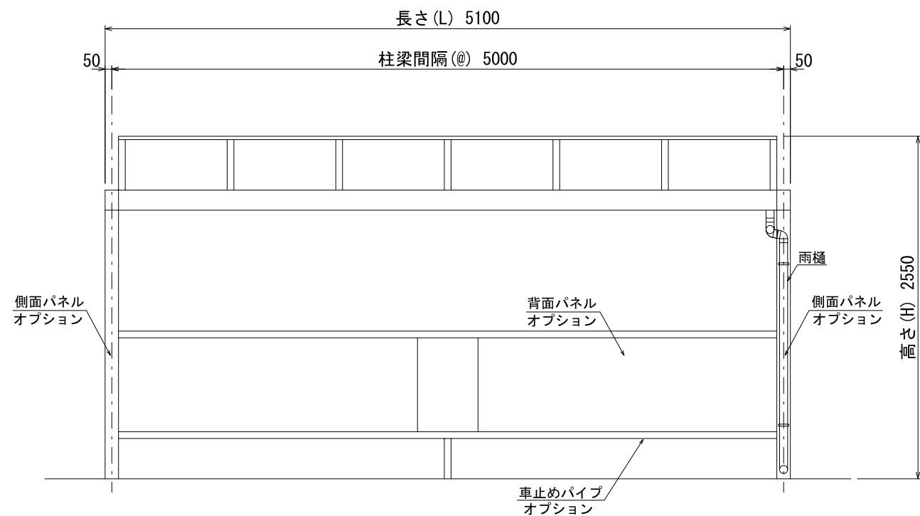
立面図
