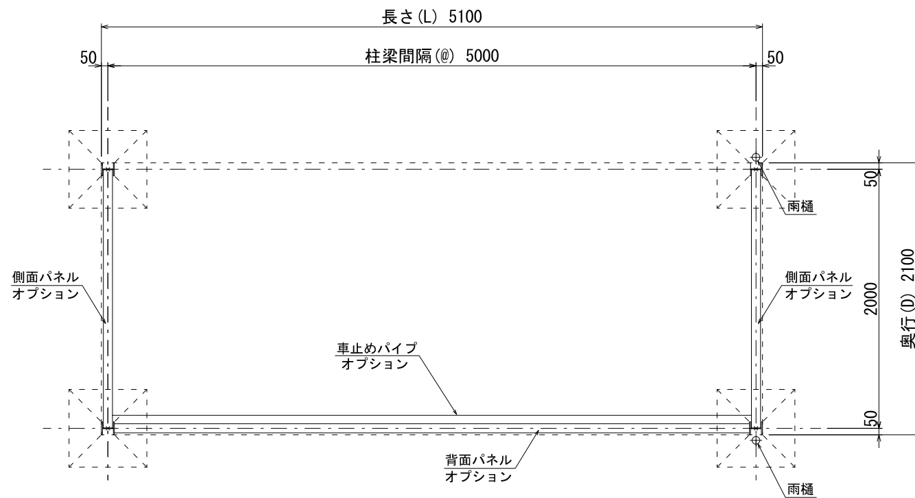
平面図
