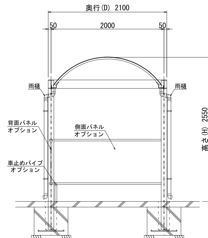
断面図
