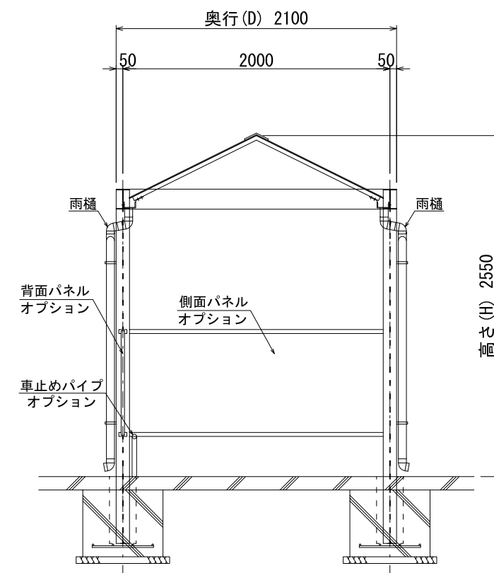
断面図
