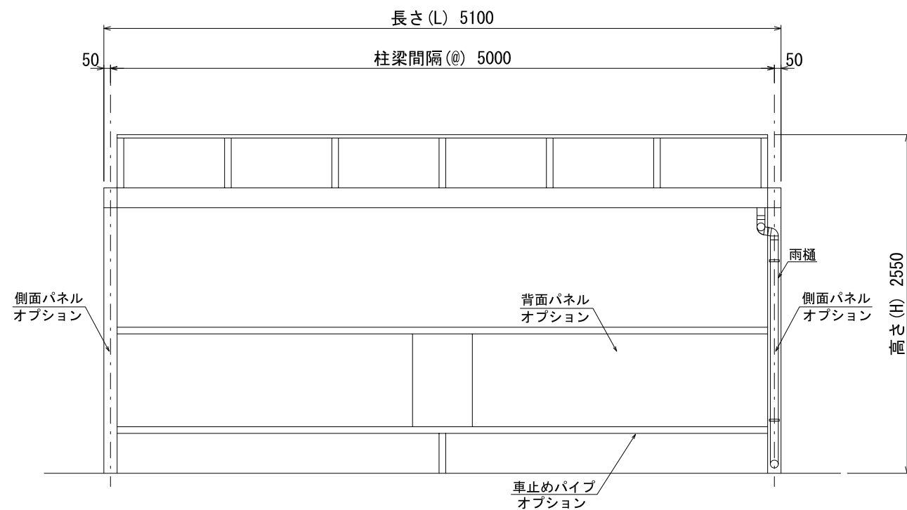
立面図
