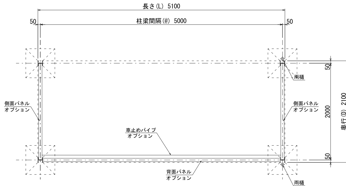
平面図
